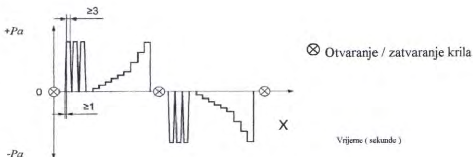
Dijagram slijeda ispitivanja propusnosti zraka
