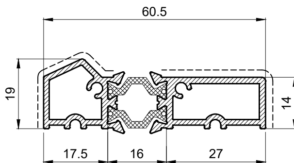
PR65241 0.879 Kg/m
