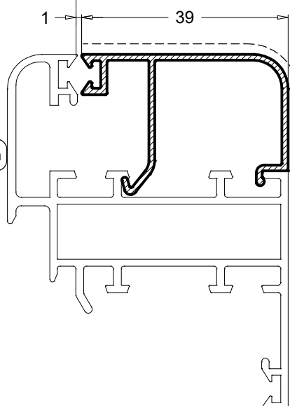
PR58567 0.332 Kg/m
