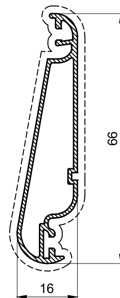
PS 01866 0,459 Kg/m
