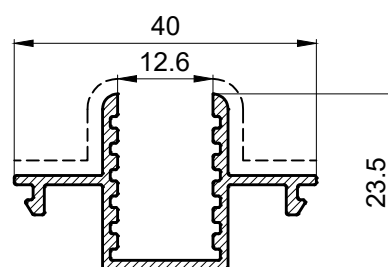
PS 03019 0,366 Kg/m
