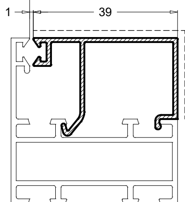
PR58567 0.332 Kg/m
