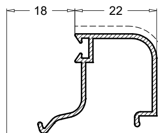
PR58558 0.273 Kg/m
