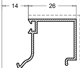
PR58555 0.280 Kg/m
