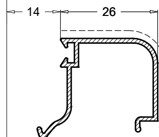
PR58556 0.270 Kg/m
