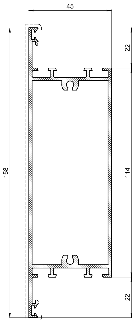
PM 40015 0,624 Kg/m
