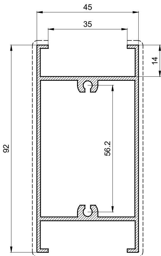
PM 40061 1,378 Kg/m
