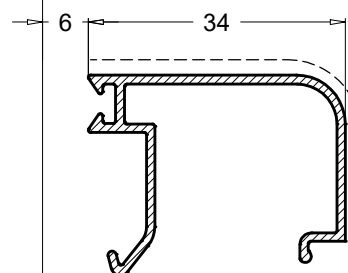
PR58552 0.295 Kg/m
