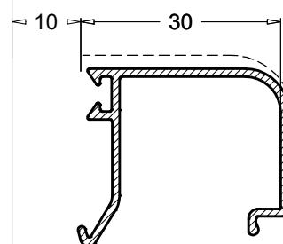
PR58554 0.281 Kg/m
