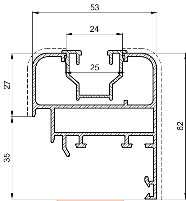
PM 40063 0,989 Kg/m
