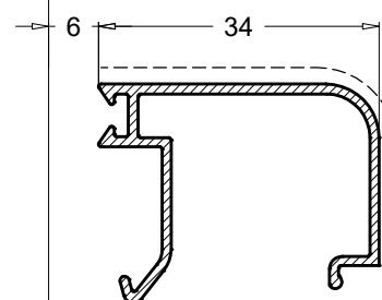
PR58552 0.295 Kg/m
