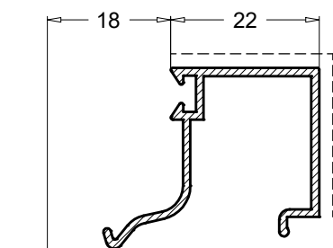
PR58557 0.276 Kg/m
