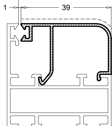
PR58567 0.332 Kg/m
