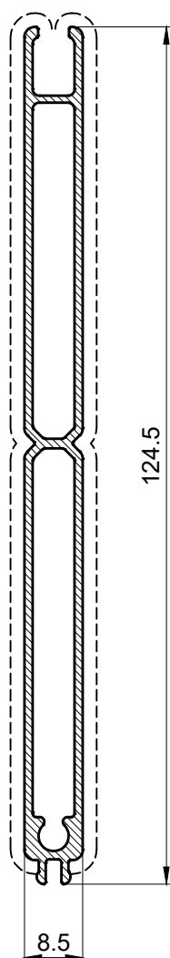
PM 50054 0,903 Kg/m
