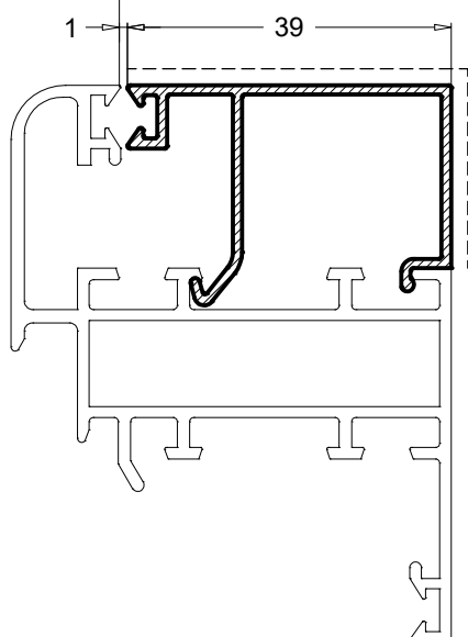
PR58567 0.332 Kg/m
