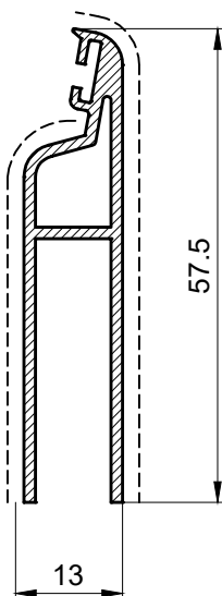
PS 15060 0,509 Kg/m
