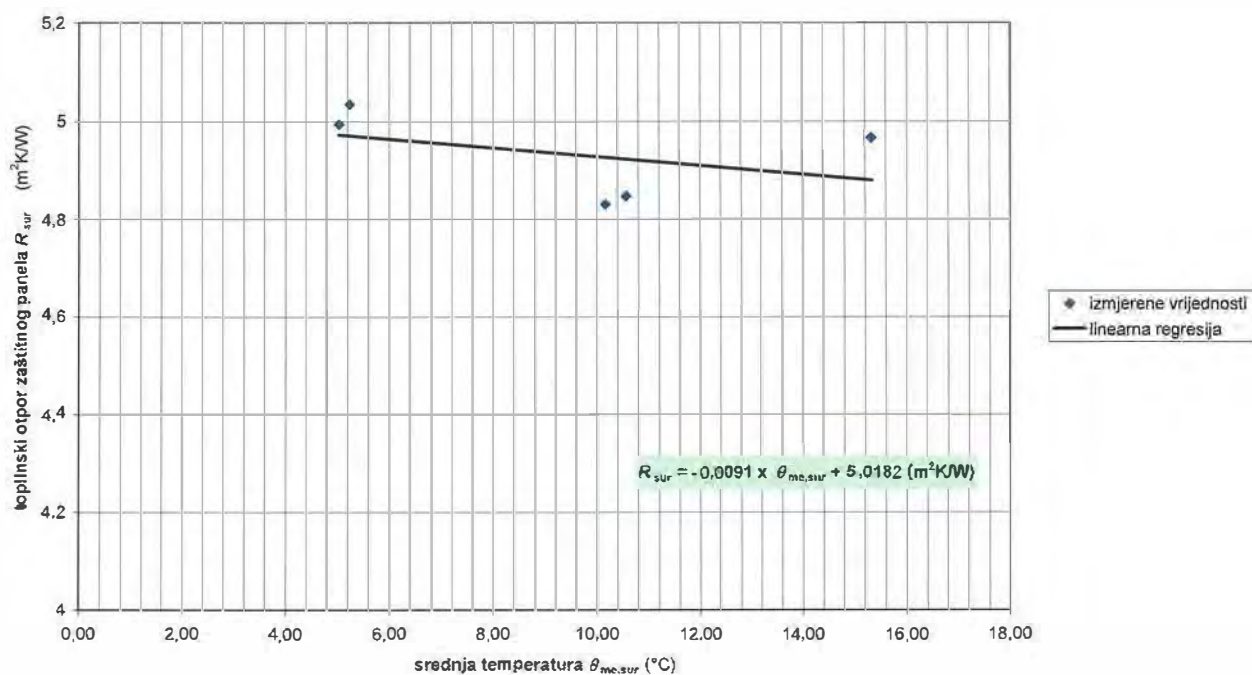
toplinski otpor zaštitnog panela
