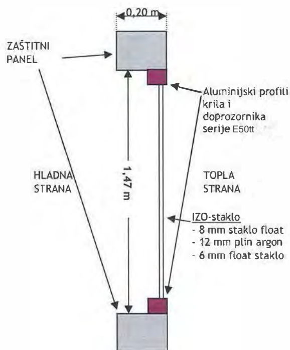
Skica mjernog složaja
