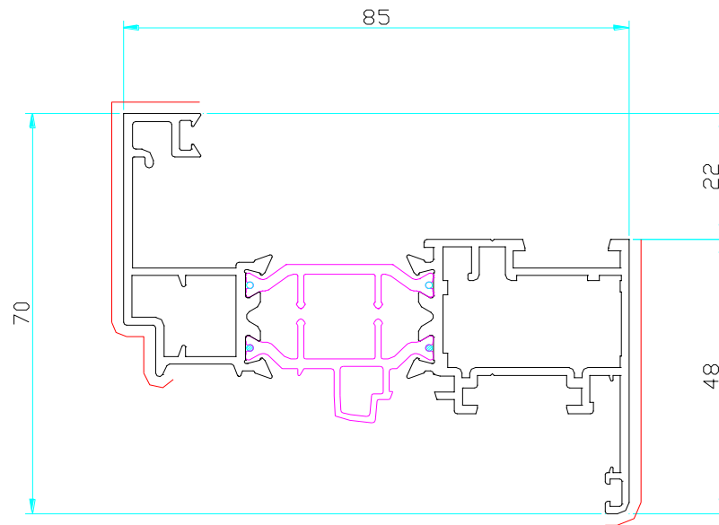
PE85110- 1.602 Kg/m
