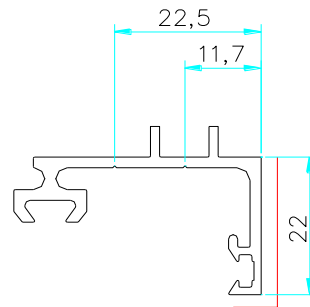
PR58539 0.430 Kg/m
