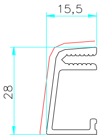
PR58541 0.310 Kg/m
