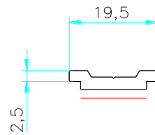
PR50550 0.160 Kg/m
